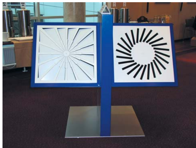
Foto 3. Nawiewniki serii FDE i VDW do pomieszczeń powyżej 2,60m i do dużych wydatków
