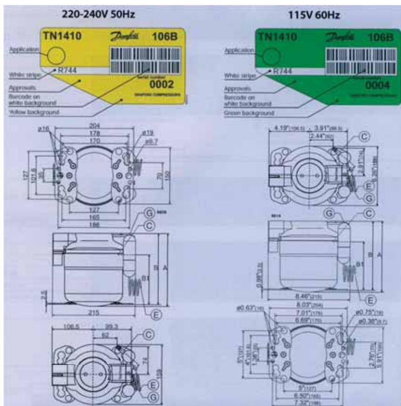
Rys. 1. Sposób oznakowania i gabaryty hermetycznych agregatów sprężarkowych firmy Danfoss, przeznaczonych do pracy z dwutlenkiem węgla
