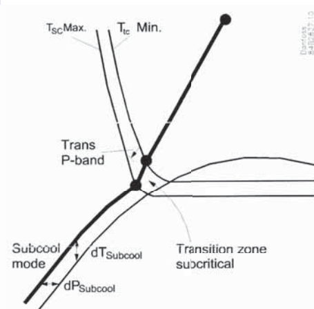
Rys. 2. Zakres regulacji ciśnienia i temperatury dwutlenku węgla za chłodnicą gazu
