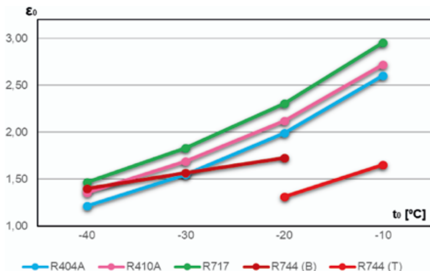
Rys. 5. Zależność współczynnika wydajności chłodniczej od temperatury parowania dla analizowanych czynników chłodniczych [opr. wł.]
